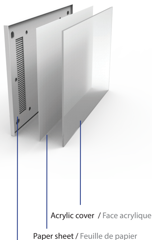
I-Sign Eco frame / Cadre I-Sign Eco
