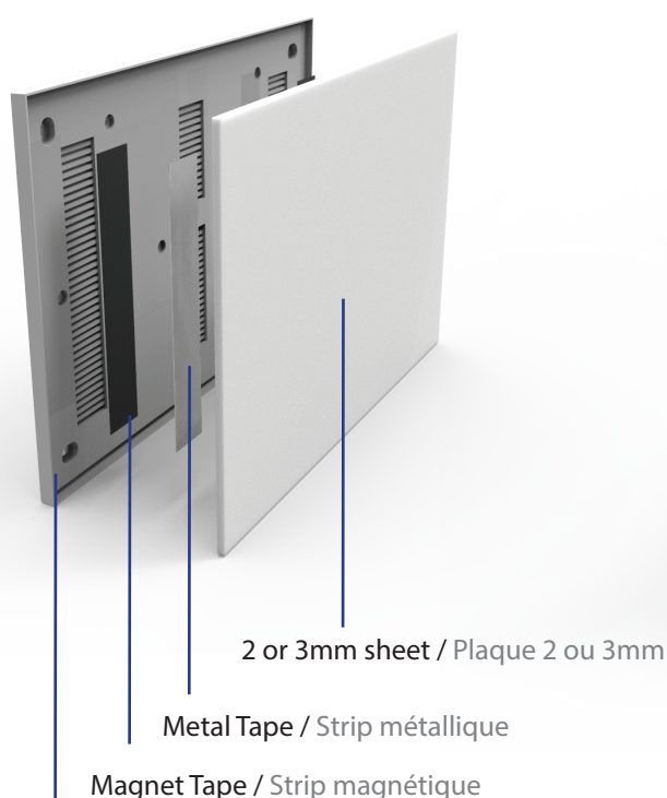
I-Sign Eco frame / Cadre I-Sign Eco
